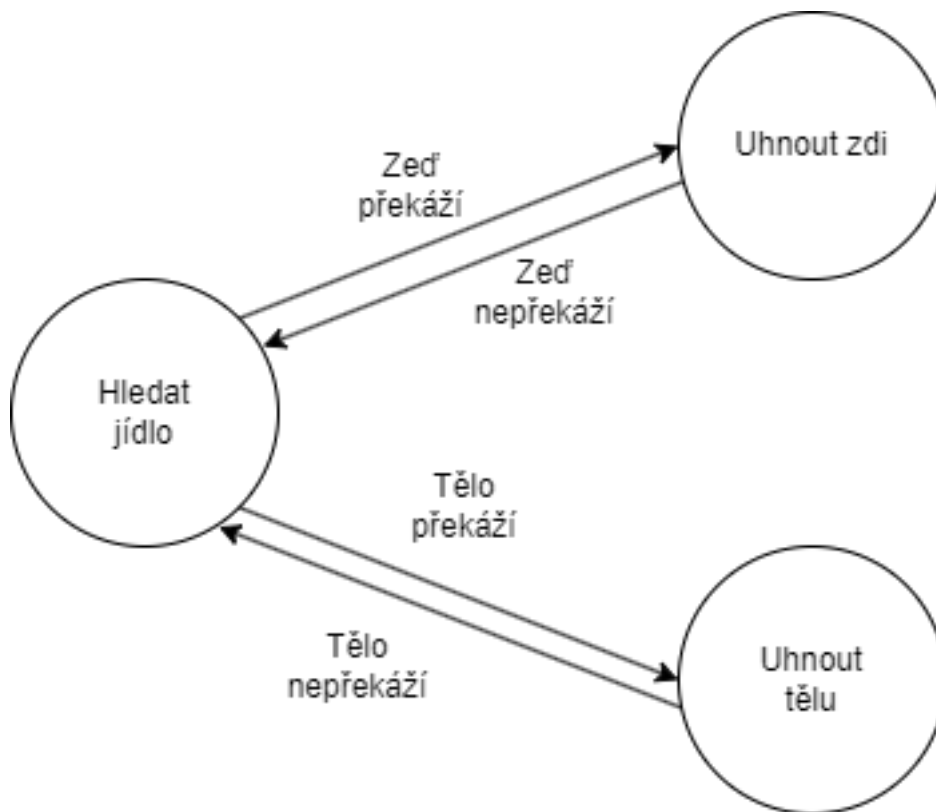
Obrázek 1.1: Příklad KA pro jednoduchou hru Snake. Obsahuje tři stavy a čtyři přechody. Had se postupně přibližuje k jídlu, ale pokud má před sebou zďď a nebo svoje tělo, tak se těmito prvky pokusí vyhnout.
